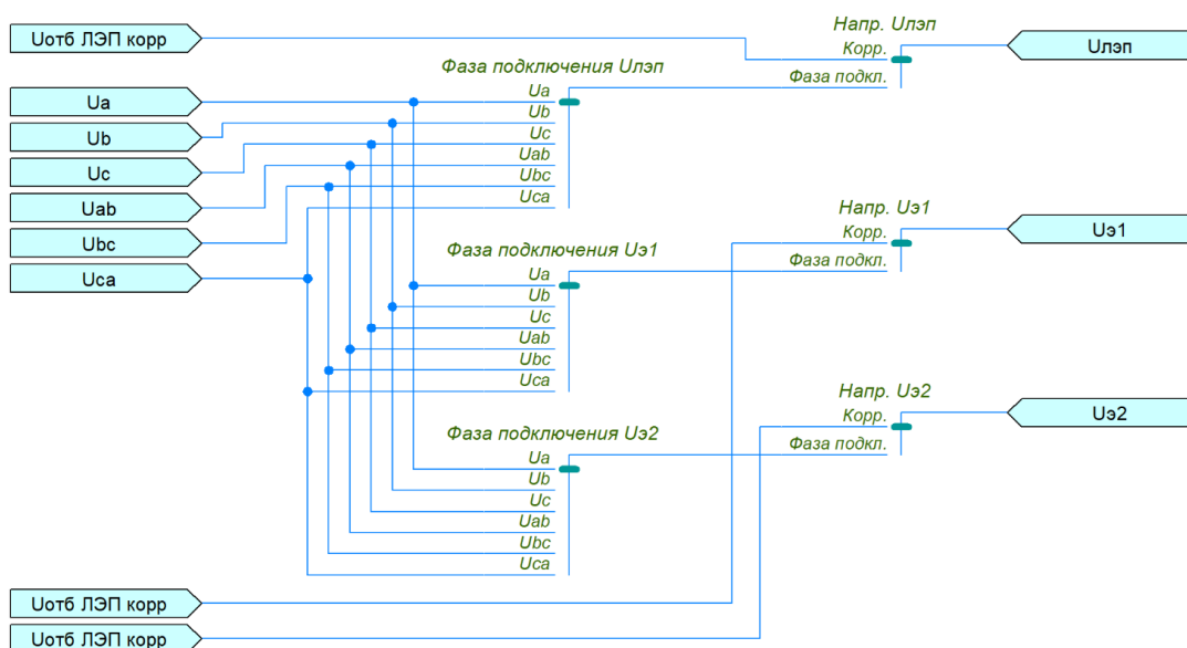
Рисунок 2.86 – Функциональная схема настройки аналоговых значений U_{лэп} , U_{э1} , U_{э2}
